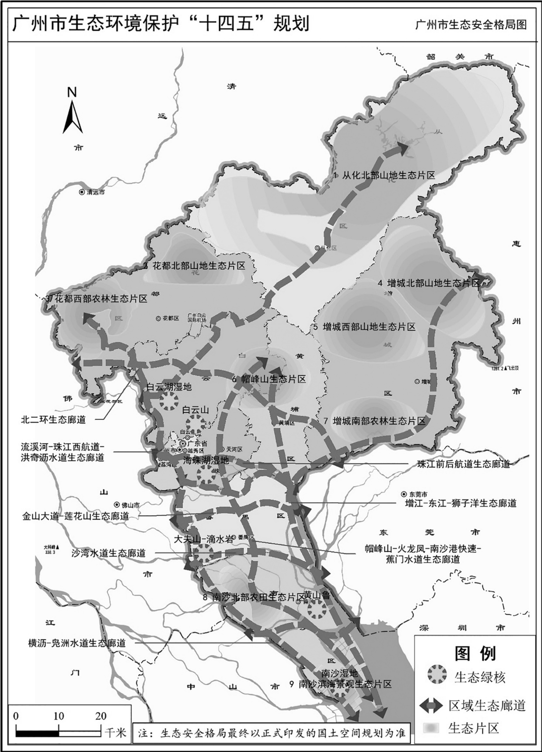
图 2 广州市生态安全格局图
