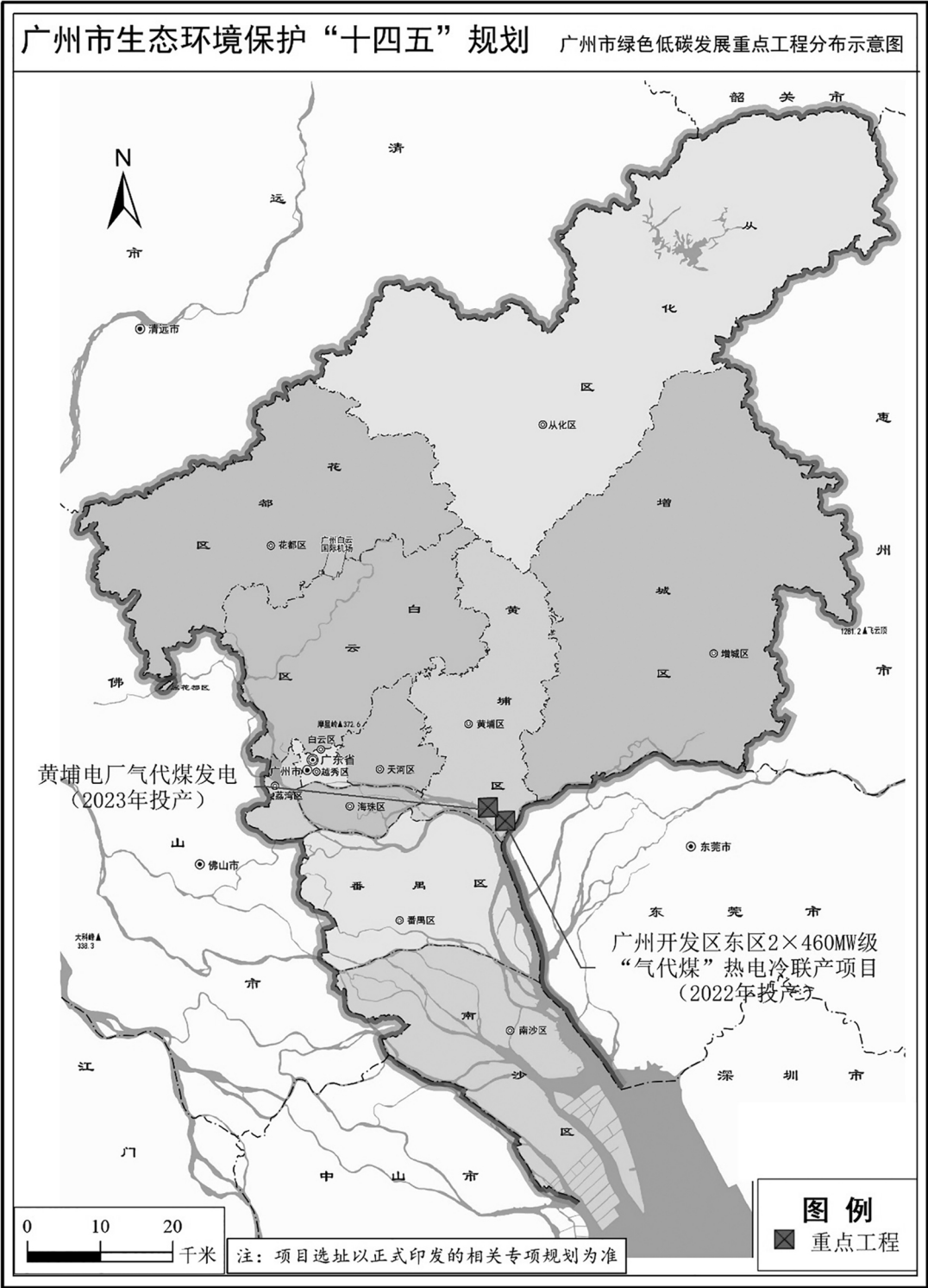
图 4 广州市绿色低碳发展重点工程分布示意图
