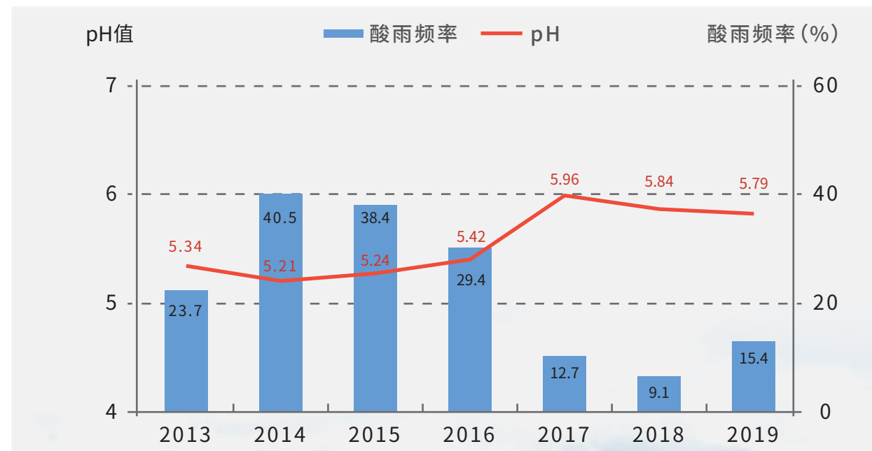
图10 2013-2019年降水pH值和酸雨频率
